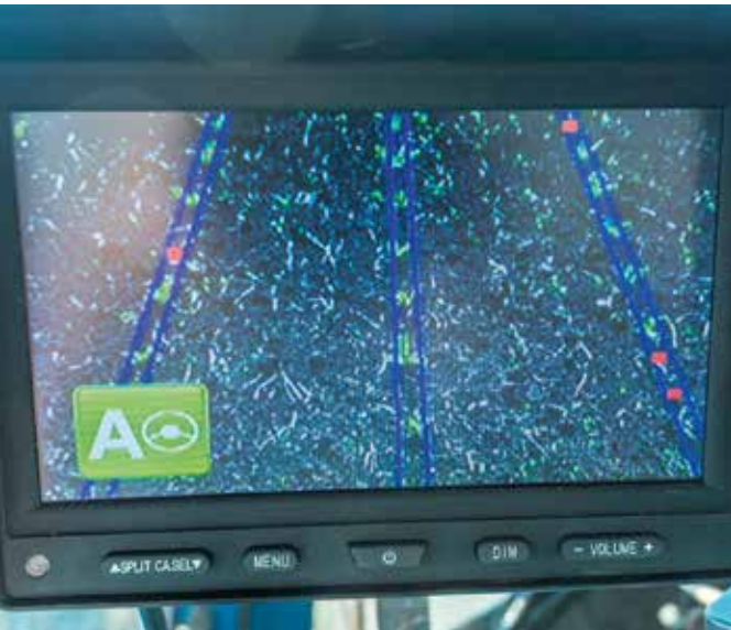
Bestandteil des Beobachtungssystems CultiCam ist ein 7"-Bildschirm, der Informationen über die Identifizierung des Bestands an das Bedienungspersonal weiterleitet.
